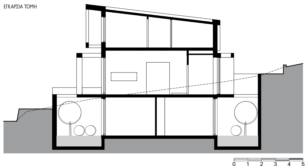
ΕΓΚΑΡΣΙΑ ΤΟΜΗ
